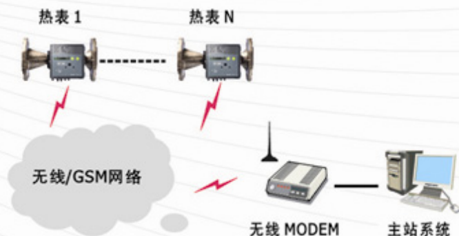
GSM/无线通讯系统图
